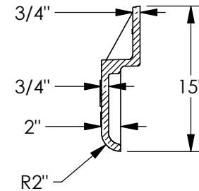
SECTION B-B SCALE 1 : 14
