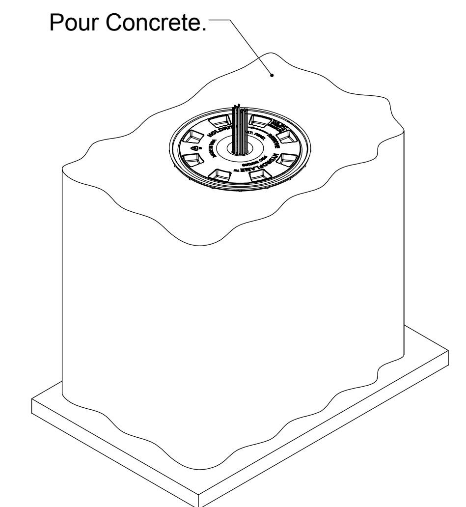
POUR CONCRETE. (Fig. 7)
