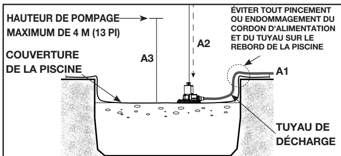
Figure A - Installation pour une piscine enterrée (vue en coupe)
