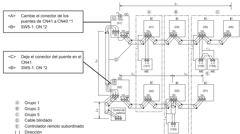
[Fig. 11.3.1] Controlador remoto M-NET
