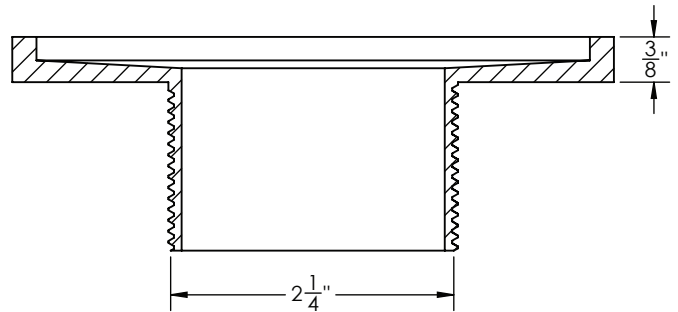
SECTION 1-1 SCALE 1 : 1
