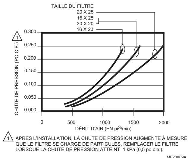
Fig. 2. Efficacité du filtre à air, chute de pression à divers débits d'air.
