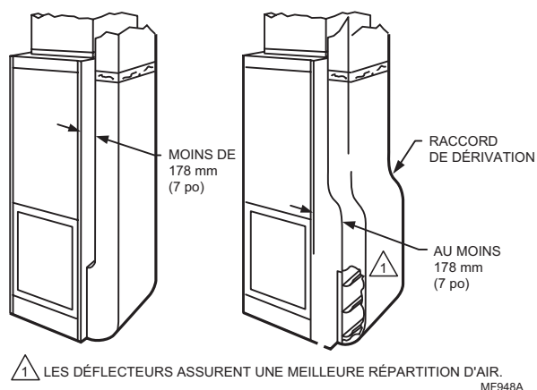
Fig. 13. Utilisation typique d'un raccord de dérivation pour assurer un dégagement suffisant au filtre à air à élément filtrant à fibres.
