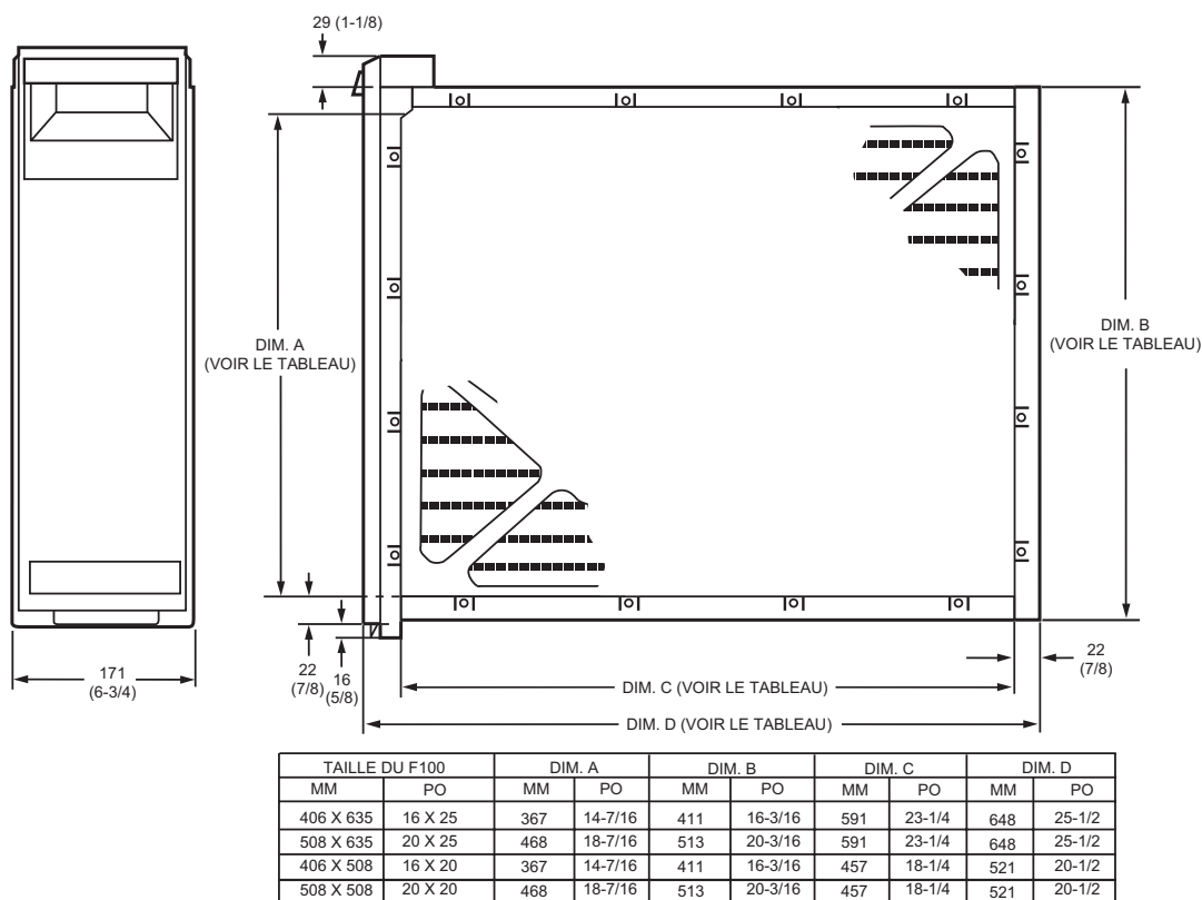
Fig. 1. Encombrement du filtre à air en mm (po).
