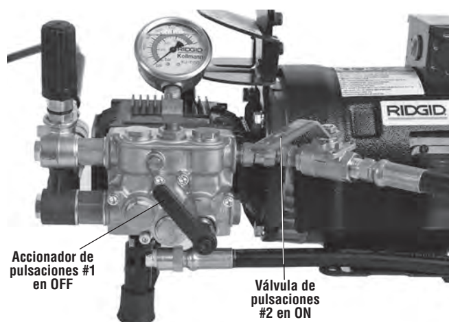
Figura 6 – Ajustes para franquear curvas y sifones
