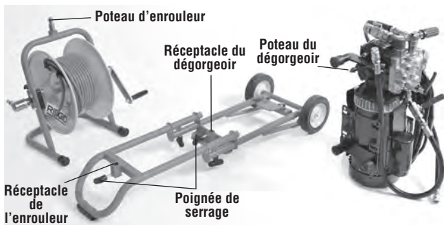
Figure 2A – Dégorgeoir haute-pression, diable H-10 et enrouleur
