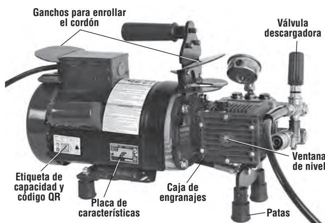
Figura 1 B – Máquina limpiadora de agua a alta presión (se muestra la KJ-1750)
