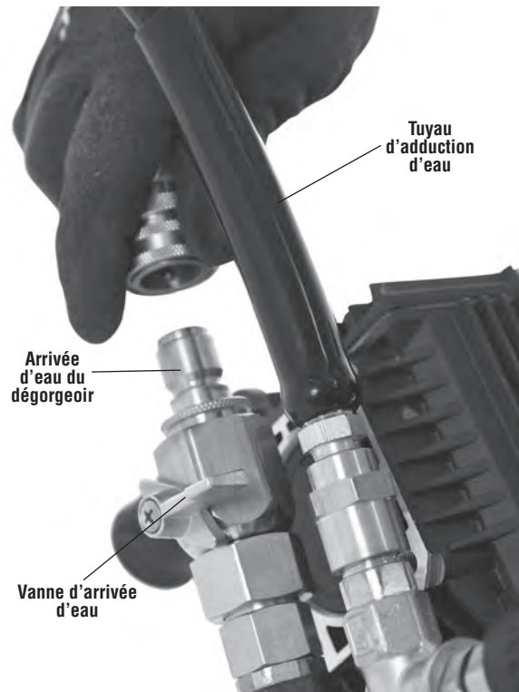
Figure 3 – Raccordement du tuyau d'adduction d'eau au dégorgeoir. Fermer la vanne d'arrivée d'eau (montrée en position fermée)
