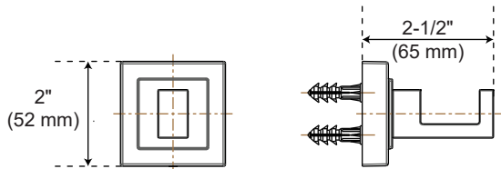
Robe Hook
