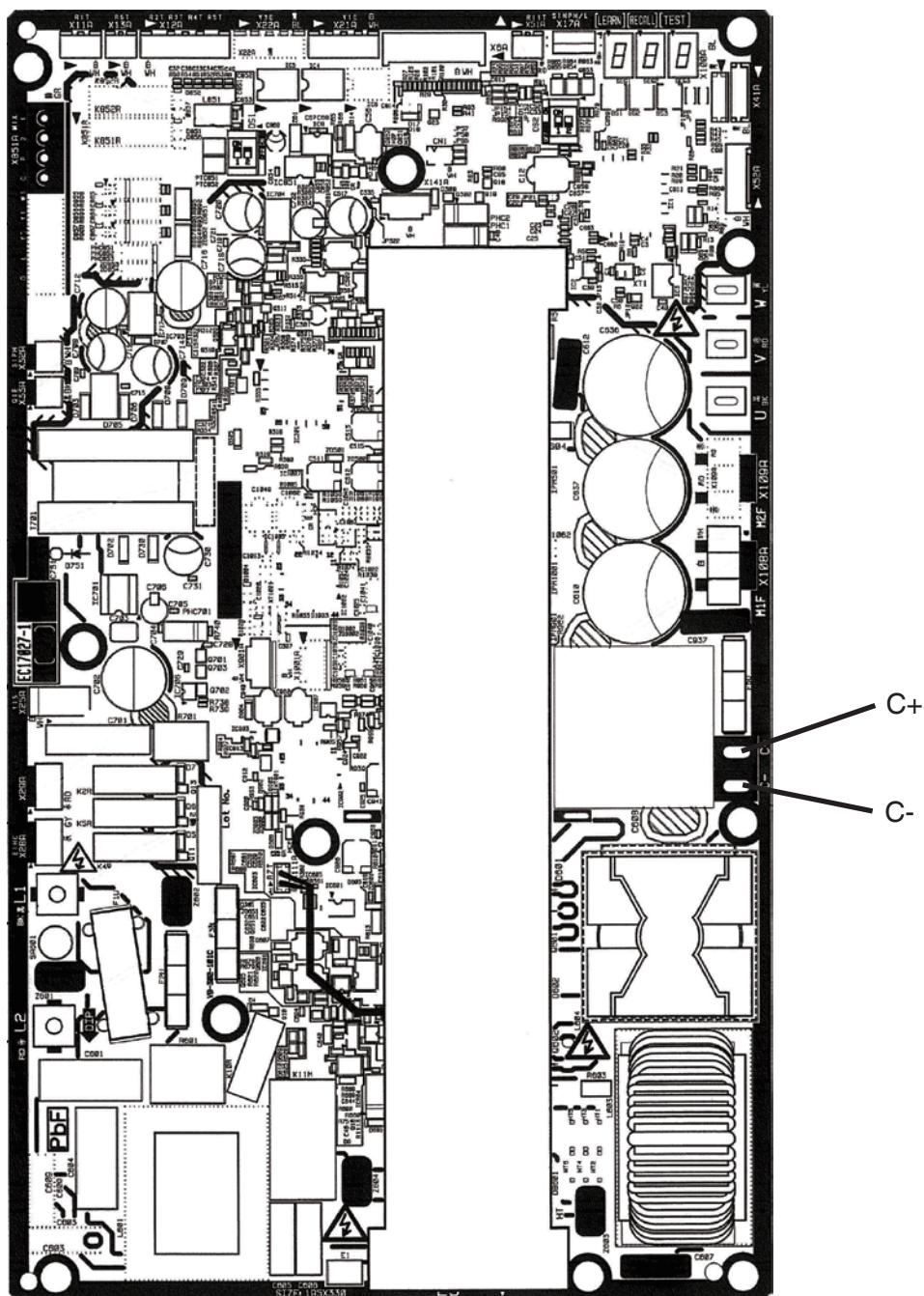
Tension du Condensateur
