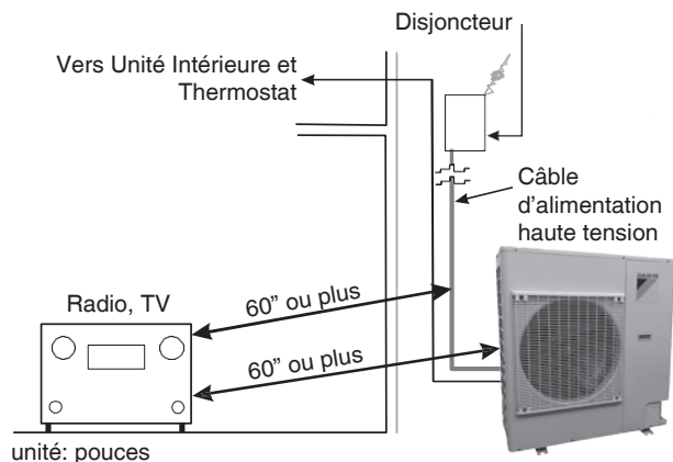
Positionnement pour Minimiser le Bruit Électronique
