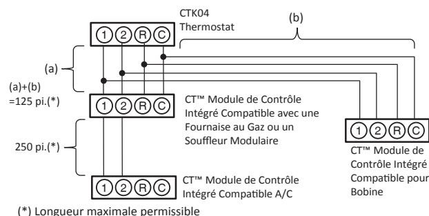
Câblage du Système (Dans le cas de CTK04)
