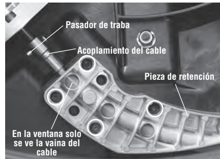
Figura 15 - Instalación de la pieza de retención del cable
