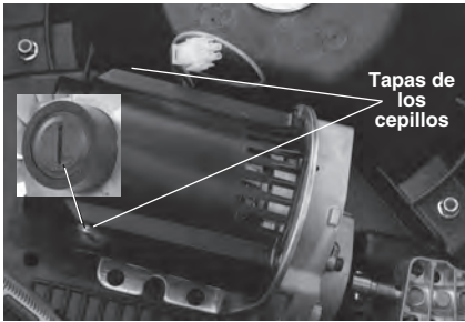
Figura 16 – Inspección y reemplazo de los cepillos del motor
