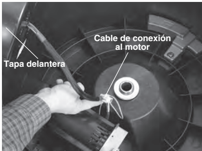
Figura 14 – Caja de la limpiadora, destapada
