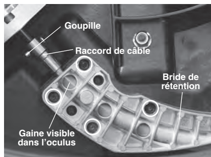
Figure 15 – Montage de la bride de rétention du câble
