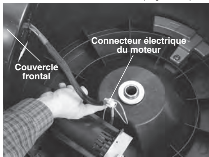
Figure 14 – Ouverture du couvercle frontal du dégorgeoir
