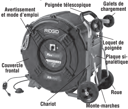
Figure 1A – Dégorgeoir RIDGID® FlexShaft
