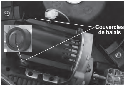
Figure 16 – Inspection et remplacement des balais moteur
