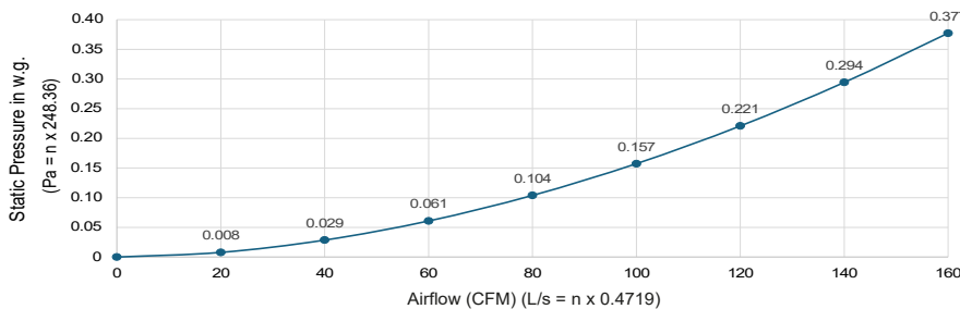
RENDIMIENTO DEL FLUJO DE AIRE A LA SALIDA
