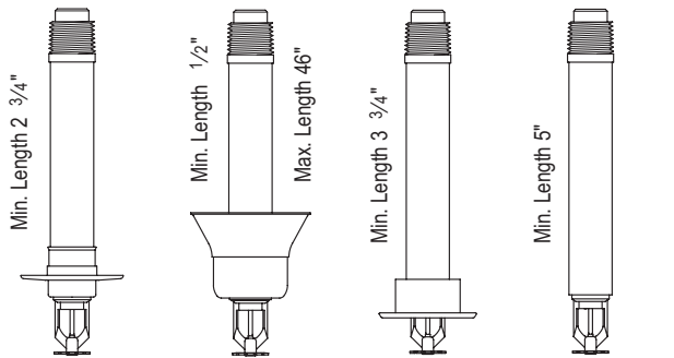
60-36X-X-XXX w/Std. Escutcheon 60-33X-X-XXX w/Deep Escutcheon 60-37X-X-XXX w/Std. Recessed Escutcheon 60-32X-X-XXX w/o Escutcheon
