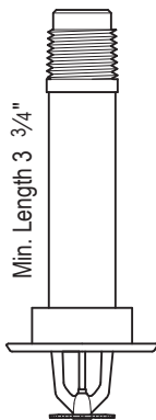
63-10X-X-XXX w/Std. Escutcheon
