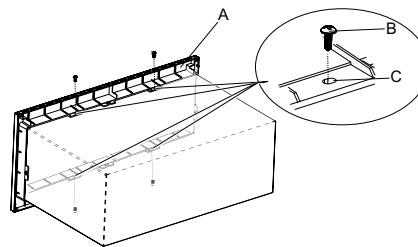
A. Cadre de garniture B. Vis à tôle à tête ronde n° 7-18x7/16 po (4) C. Trous de vis (4)
