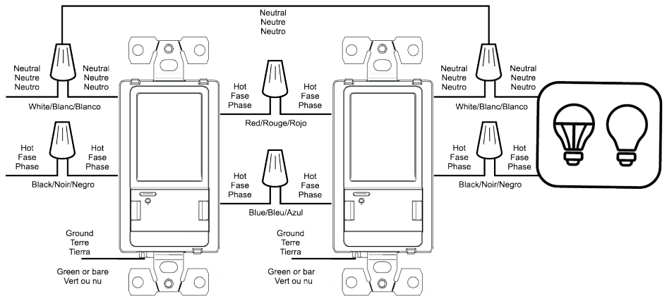
Wiring Diagrams Schema de cablage Diagrama de Alambrado
