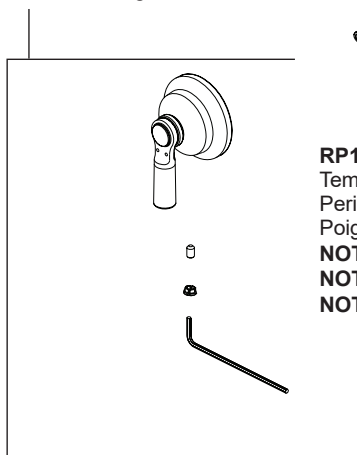
RP102146▲ Handle, Set Screws, Buttons & Wrench Manija, Tornillos de ajuste, botones y Llave Poignée, Vis de calage, boutons et Clé
