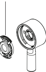
RP32102 Rotational Limit Stop Tope para Limitar Butée Rotative
