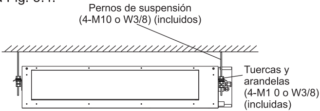
Fig. 3.4 Instalación de la unidad interior
