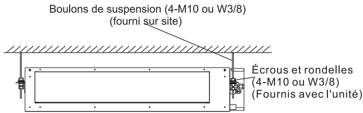
Fig. 3.4 L'installation de l'unité intérieure
