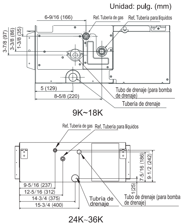
Fig. 4.1 Las posiciones de conexión de la tubería
