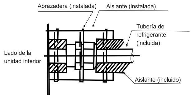
Fig. 4.4 Procedimiento de aislamiento de tuberías
