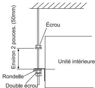
Fig. 3.5 Boulons de suspension et écrous
