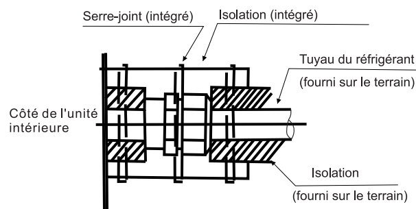
Fig. 4.4 Procédure d'isolation de la tuyauterie
