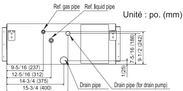
Fig. 4.1 Les positions de connexion du tuyau
