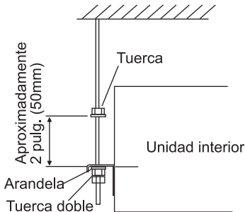
Fig. 3.5 Pernos de suspensión y tuercas
