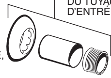
M970738-0070A ASSEMBLAGE DU DIAPHRAGME, DÉBITS RESTANTS
