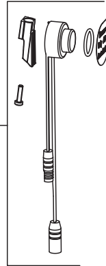
M970734-0070130A ASSEMBLAGE DU CAPTEUR POUR URINOIR FV, 0,125 GPC
